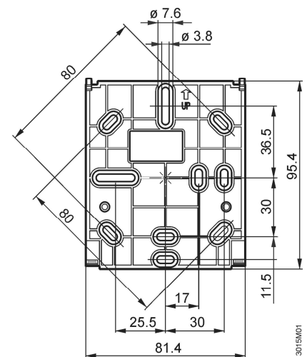
Baseplate
