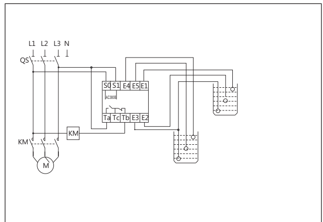
Для НЈУW1-BL1, НЈУW1-BL2 напряжение питания 380V
