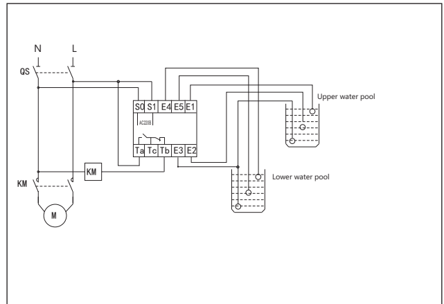
Для НЈУW1-BL1, НЈУW1-BL2 напряжение питания 220V
