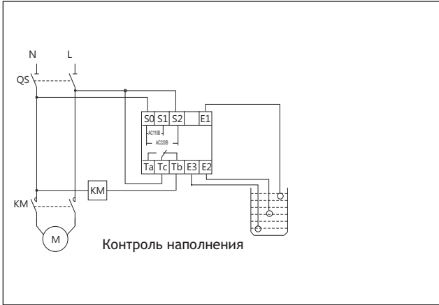
Для НЈУW1-NL1, НЈУW1-NL2 напряжение питания 110V/220V
