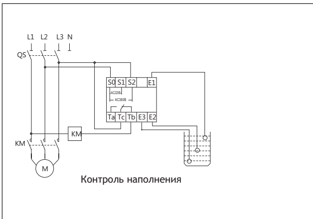
Для НЈУW1-NL1, НЈУW1-NL2 напряжение питания 220/380V
